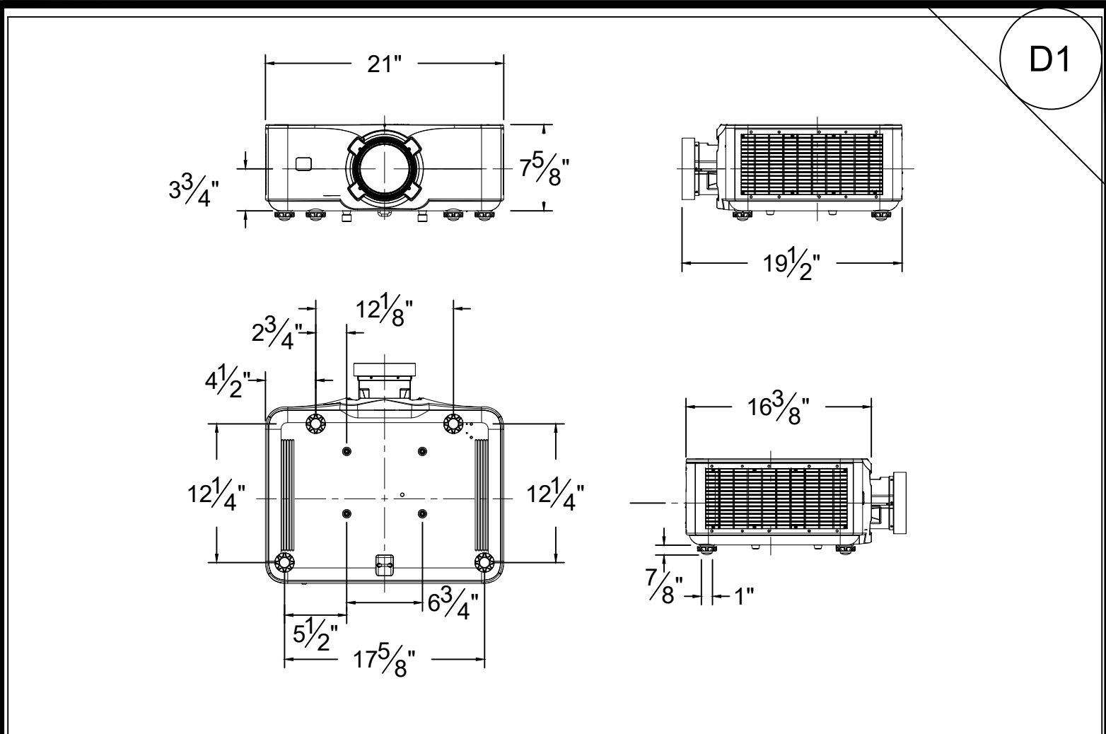
CHRISTIE 4K1000-KS
