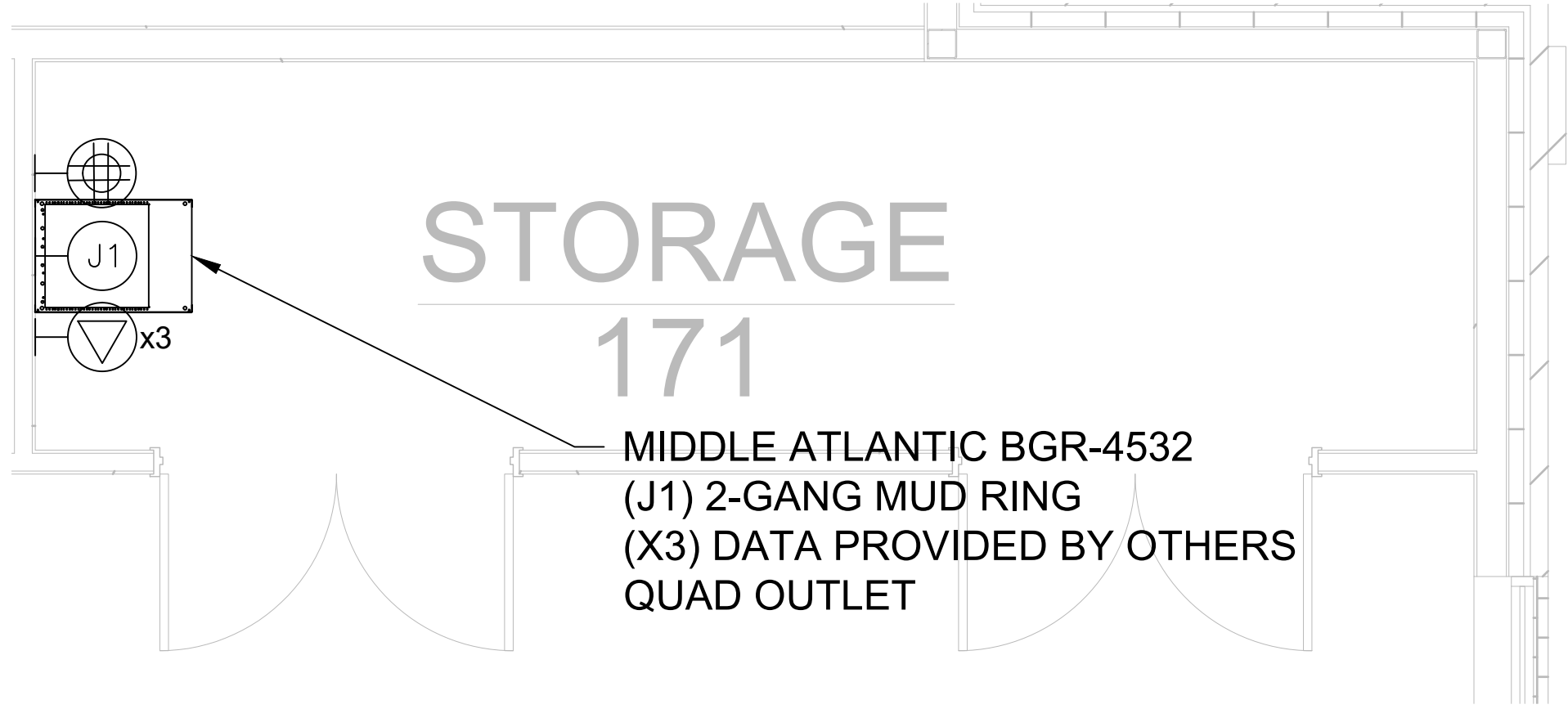
1 AV RACK CLOSET (STORAGE 171) SCALE: 3/8"=1'-0" ARCH D
