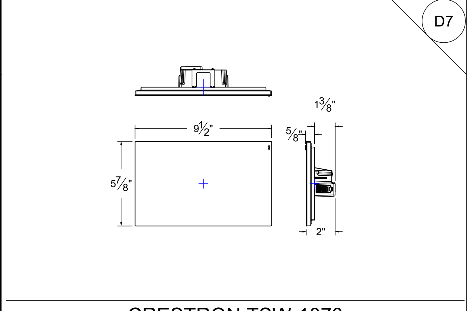
CRESTRON TSW-1070
